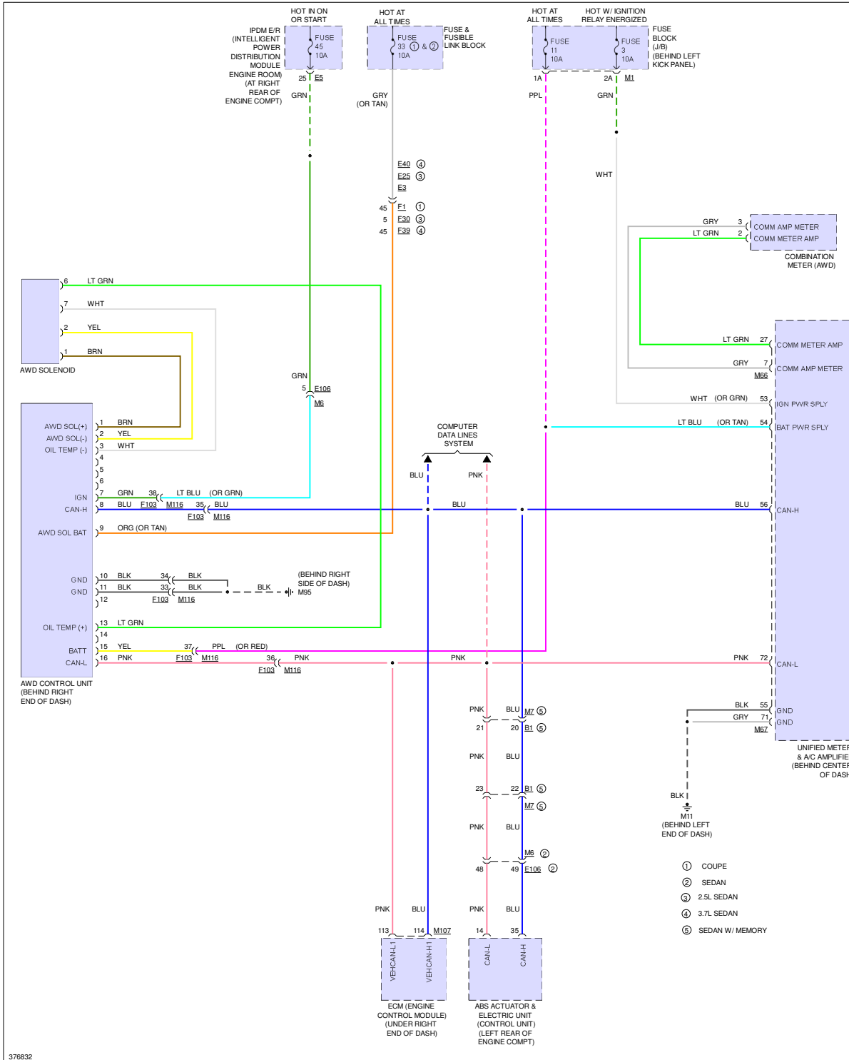
Fig 2: AWD Circuit
